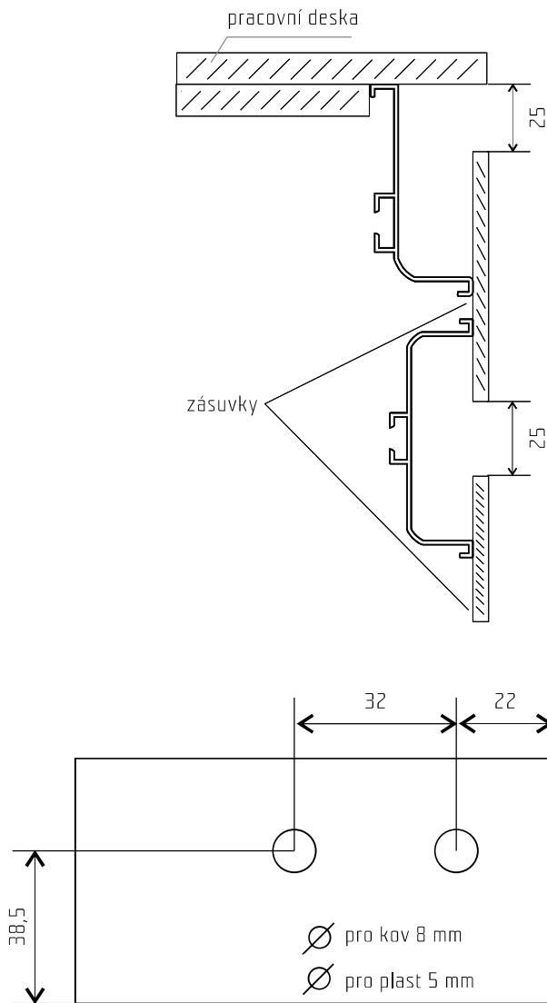
Spojka pro profil C a J
