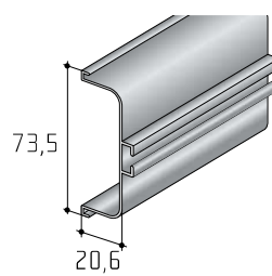
Profil C kování
