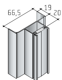
Profil vertikální k C a J
