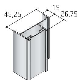
Profil vertikální hranový
