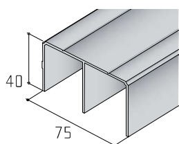
Profil S05
