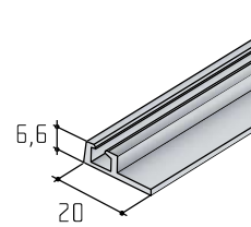
Profil S06 N-1
