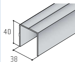
Profil S05-1
