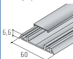
Profil S06 NN krycí profil S06 N
