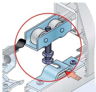
Montáž vozíku
