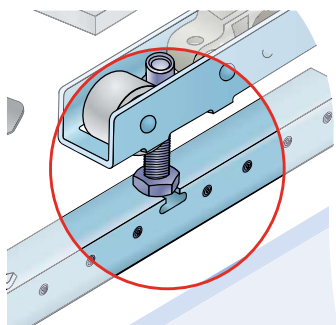
Montáž vozíku – nový úchyt
