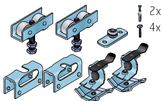
Sada S80 Frame 65 (pro dveře z rámu S65)
