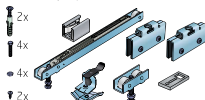
Sada S80 Glass SC s tlumičem, pro posuvné skleněné dveře*
