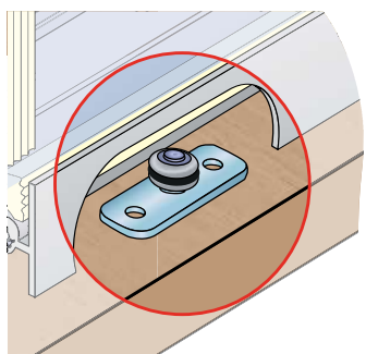
Detail spodního vedení
