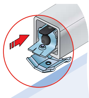
Detail garnýže – úchyt AL lišty boční
