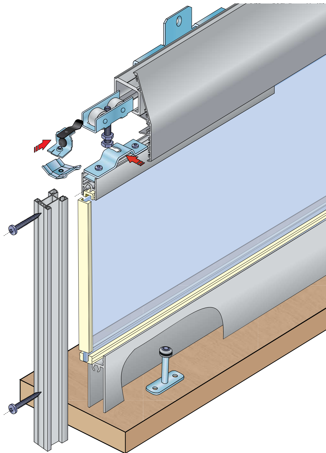
Sada S80 Frame SC (pro dveře z rámu S55)
