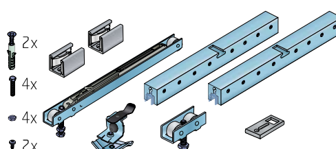
Sada S80N Glass SC N (pouze pro kalená skla do 45 kg)
