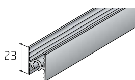
Profil S55 horní a střed.
