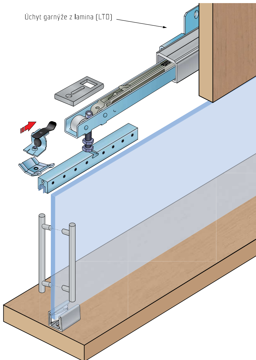
Sada S80 Glass SC s tlumičem, pro posuvné skleněné dveře*
