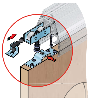
Detail montáže do stropu
