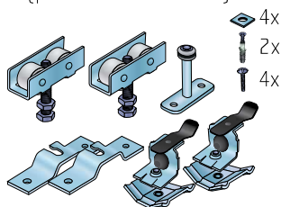
Sada S80 Frame (pro dveře z rámu S55)
