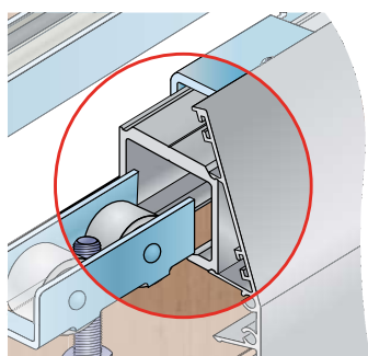
Detail montáže na bok
