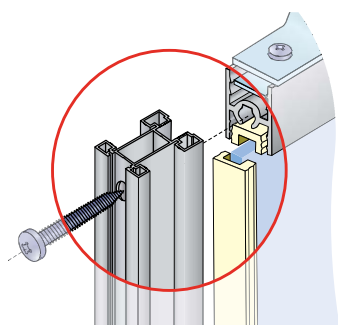
Montáž madla
