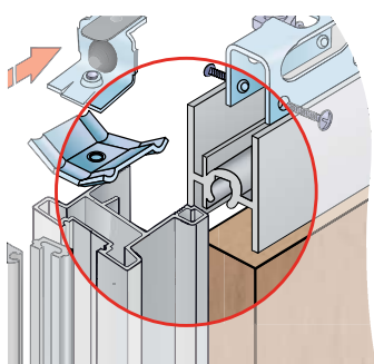
Montáž madla
