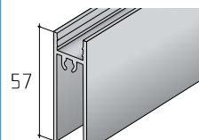
Profil S55 dolní
