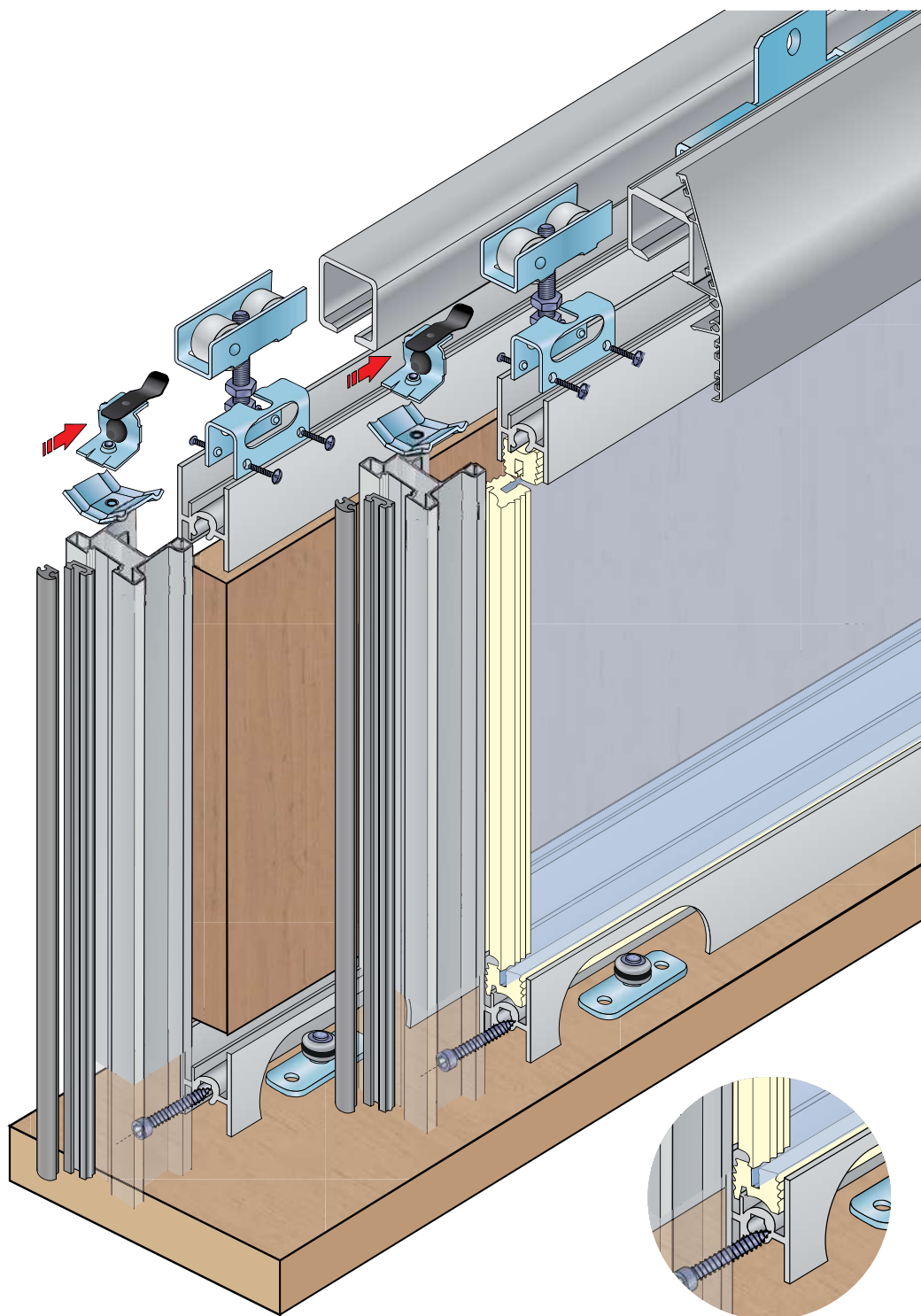
Sada S80 Frame SC (pro dveře z rámu S65)
