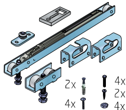
Sada S80 Frame SC (pro dveře z rámu S65)
