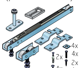
Sada S80 Frame SC (pro dveře z rámu S55)
