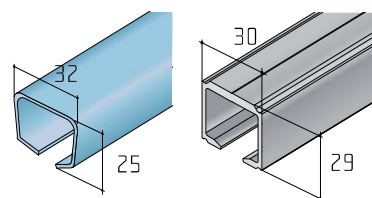
Profil S40/S80 ocel Profil S40/S80N AL
